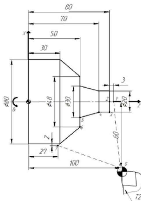
Рисунок 1. Эскиз расчетно-технологической карты
